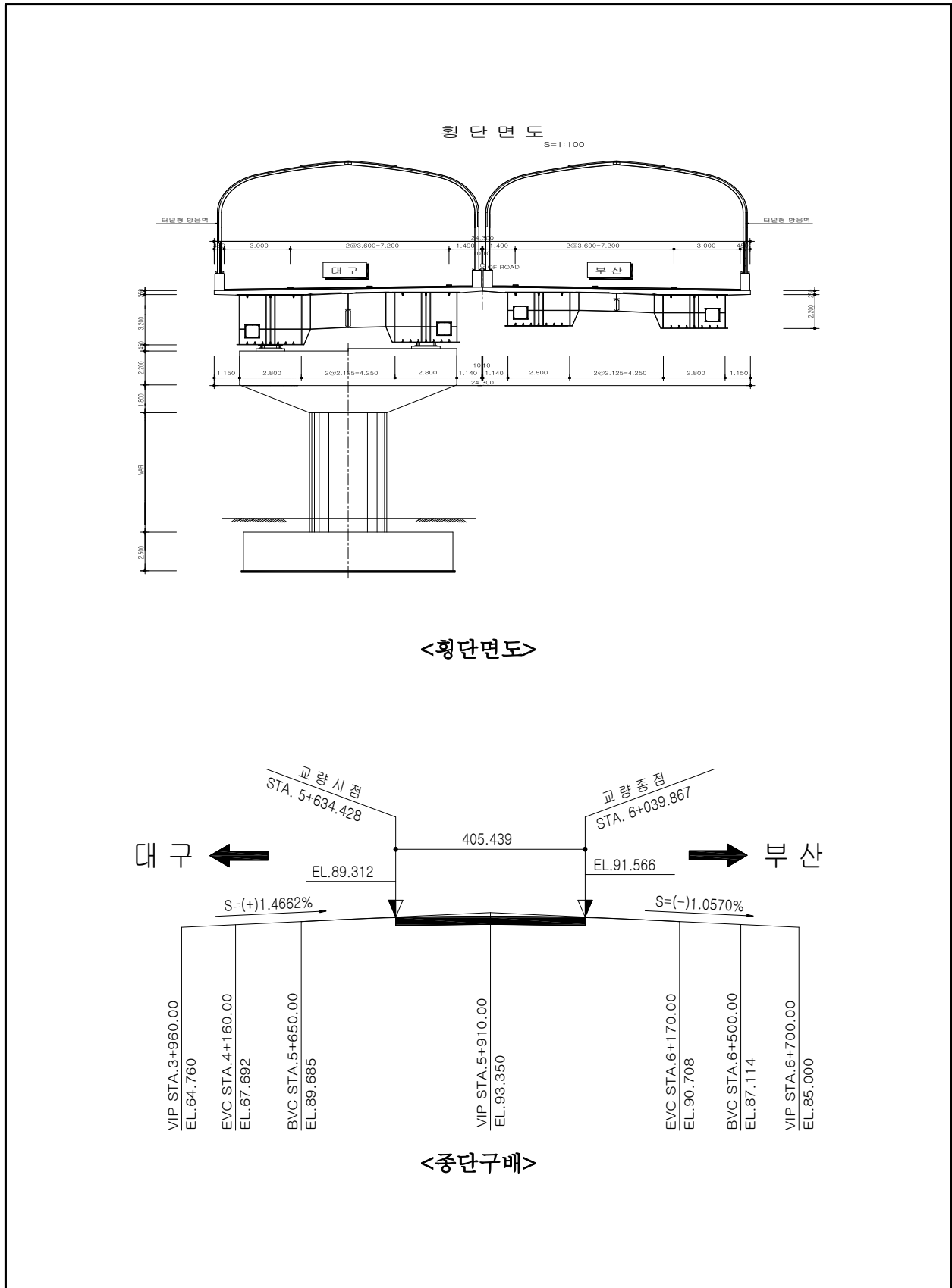
【그림 1.4.6】 노변교(부산) 횡단면도 및 종단구배
