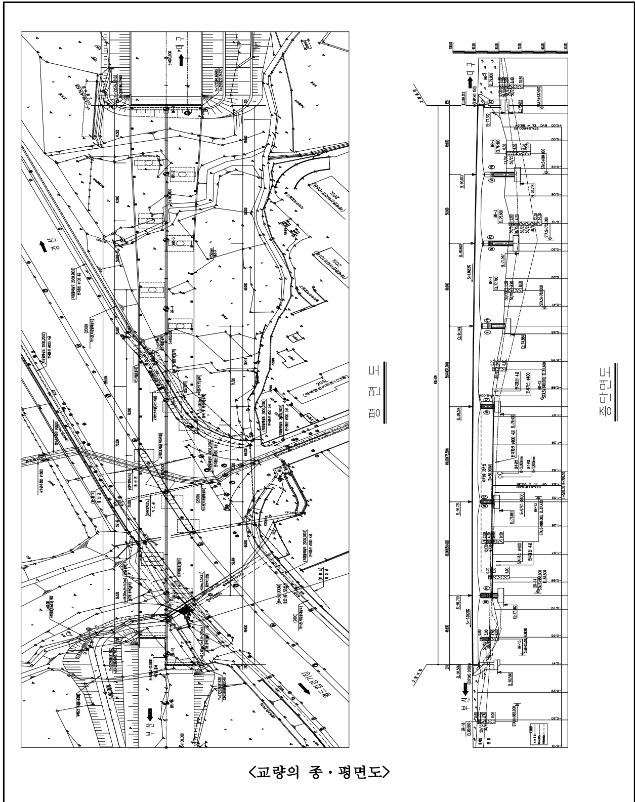
【그림 1.4.5】 노변교(부산) 종·평면도
